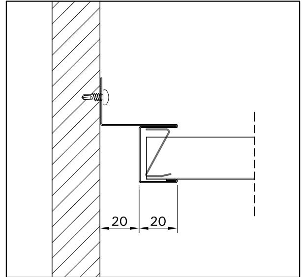
Profile W1
